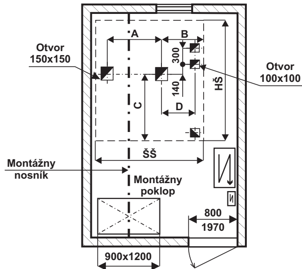
Pôdorys strojovne Typ - ATB, ATP
