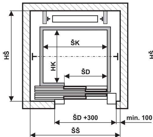
Pôdorys šachty Typ - ATZ
