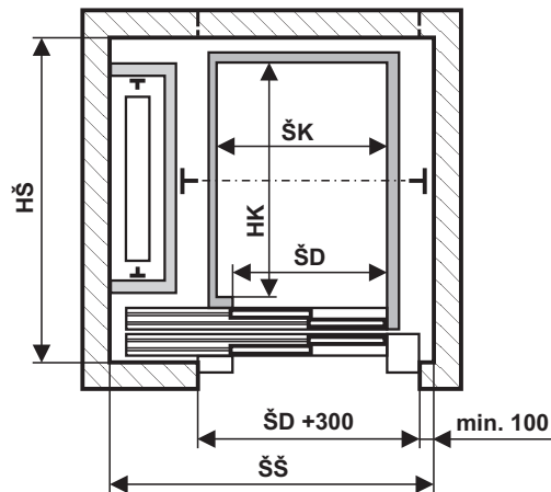
Pôdorys šachty Typ - ATB, ATP
