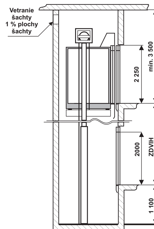
Rez šachty
