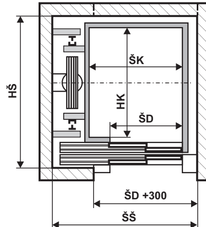
Pôdorys šachty Typ - ATB, ATP
