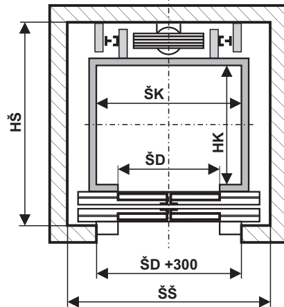
Pôdorys šachty v spodnej stanici Typ - ATB, ATP
