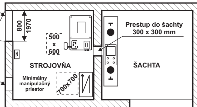
Pôdorys strojovne Typ - MZ, MB, MP
