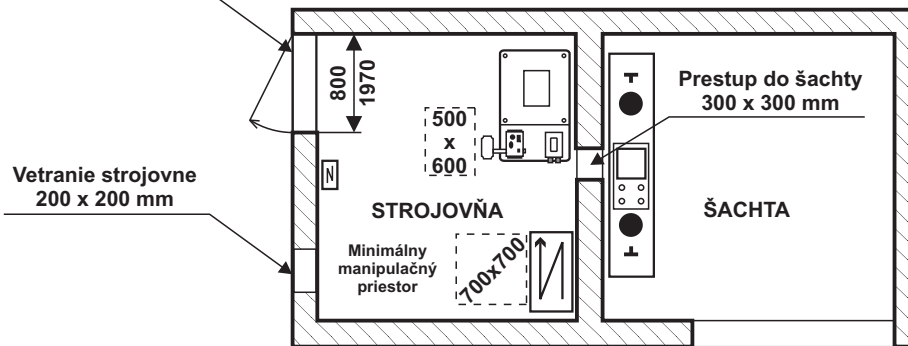
Pôdorys strojovne Typ - MZ, MB, MP
